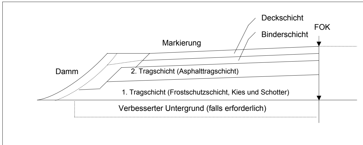
Abbildung 1: Aufbauvariante Standard
