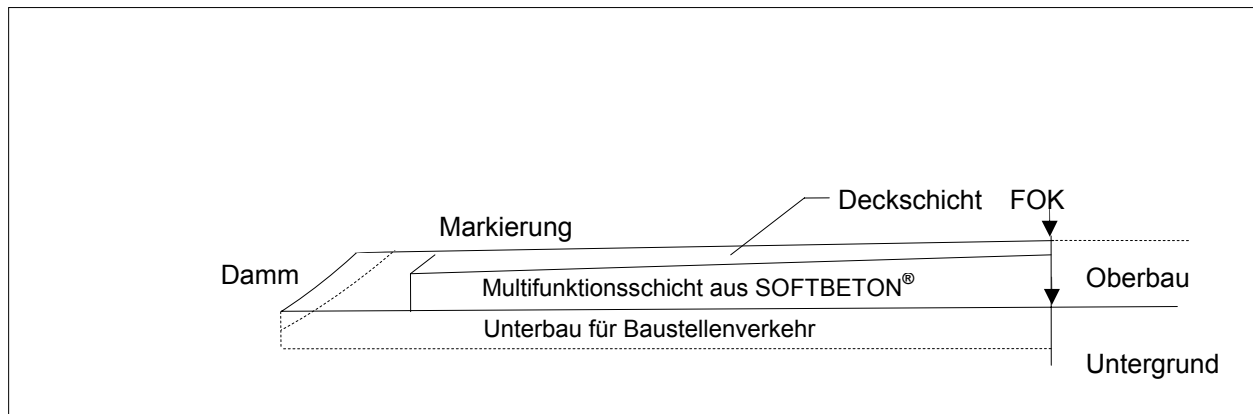
Abbildung 2: Aufbauvariante SOFTBETON®
